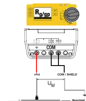
Messung: R_G Ableitwiderstand zu Schutzerde
