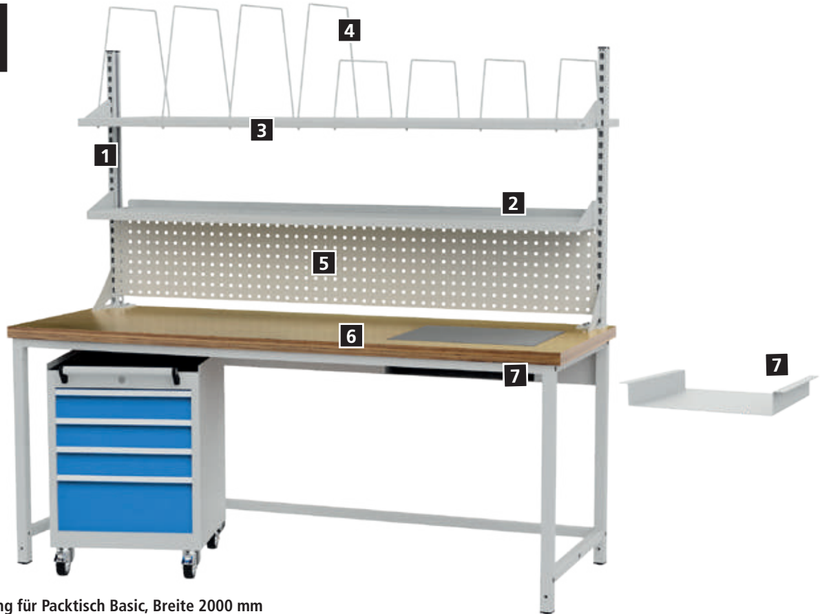
Zusammenstellung für Packtisch Basic, Breite 2000 mm
