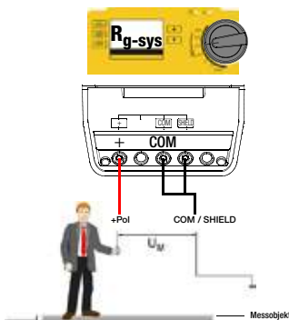
Messung: R_{G\text{-system}} Personenableitwiderstand (Mensch/Schuhe/Boden) zu Schutzerde
